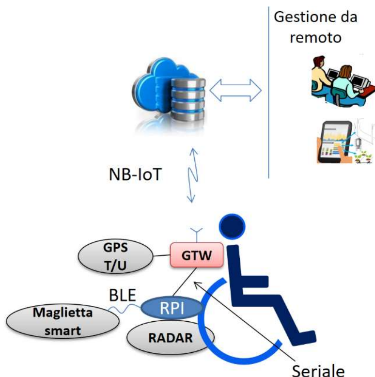
Figura 3. Architettura della carrozzina elettricamente tecnologicamente avanzata
