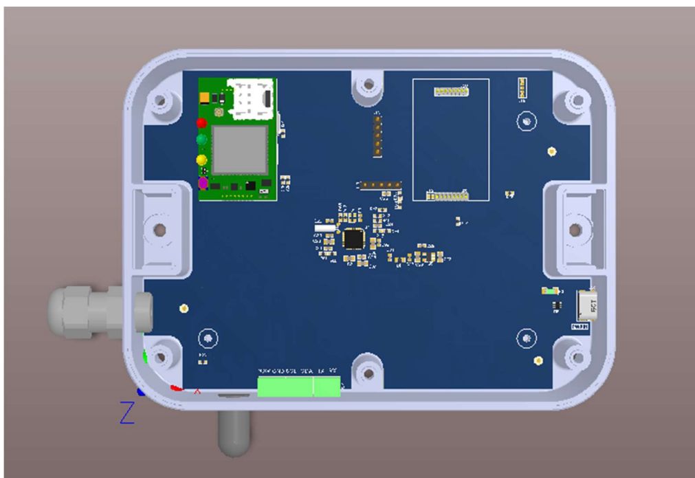
Figura 8. Hardware realizzato inserito nella meccanica di riferimento
